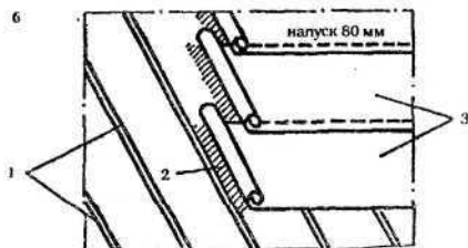
Рис. 5. Покрытие стальных кровель рулонными материалами: а — рядами параллельно коньку; б — рядами перпендикулярно коньку; 1 — прижимные гребнистаячих фальцев; 2 — горячий битум; 3 — рубероид
